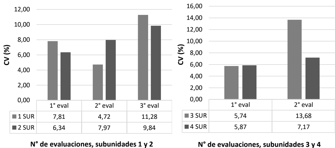
Figura 4. Representación del CV en las cuatro subunidades de riego (cañahua y cebolla).
