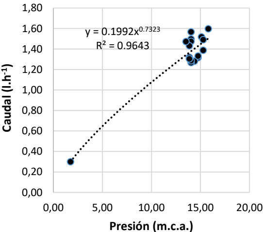
Curva de gasto en la subunidad.
