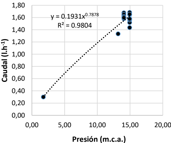
Curva de gasto en la subunidad.
