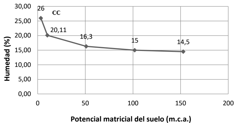
Figura 6. Curva de retención de humedad para el suelo FYL.
