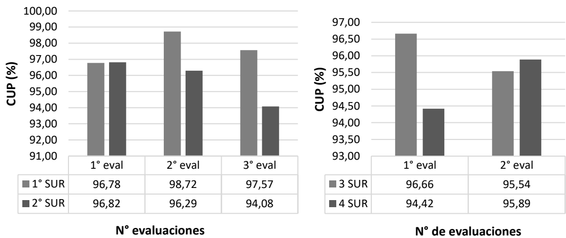
Figura 5. Representación de CUP de las evaluaciones dentro de las cuatro subunidades de riego.
