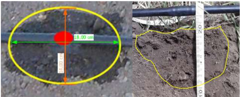
Figura 8. Formación del diámetro de mojado y bulbo húmedo.
