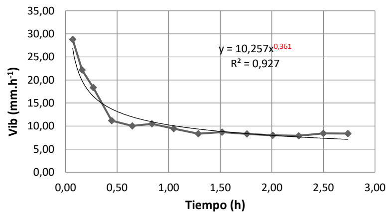
Figura 7. Curva de la velocidad de infiltración básica del suelo
