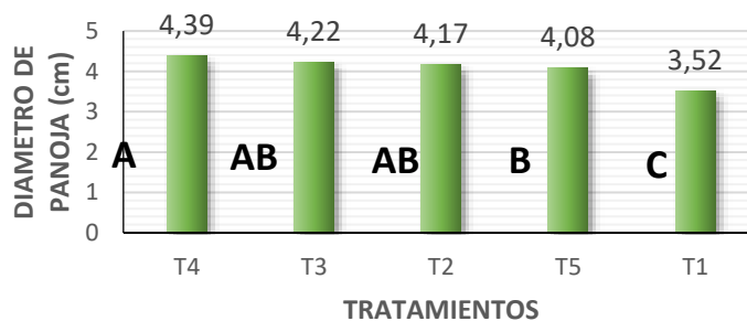
Figura 2. Prueba de Tukey al 5% para diámetro de panoja.
