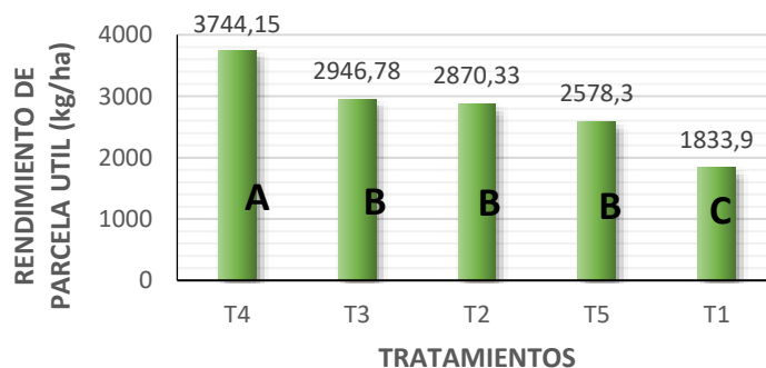
Figura 8. Prueba de Tukey al 5 % para rendimiento de parcela útil.
