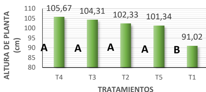
Figura 1. Prueba de Tukey al 5% para altura de planta a la madurez.
