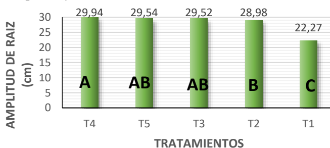
Figura 5. Prueba de Tukey al 5% para amplitud de raíz.
