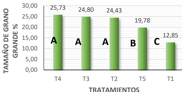
Figura 9. Prueba de Tukey al 5% para tamaño de grano grande.
