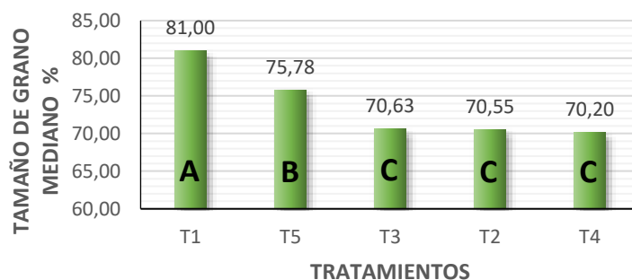
Figura 10. Prueba de Tukey al 5% para tamaño de grano mediano.
