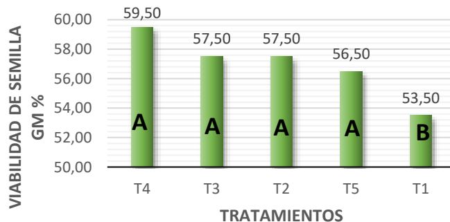
Figura 12. Prueba de Tukey al 5% para viabilidad de semilla de tamaño mediano a las 16 horas de prueba.
