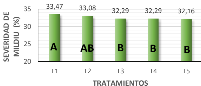
Figura 6. Prueba de Tukey al 5% para severidad de mildiu.
