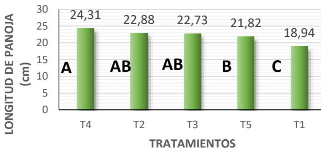
Figura 3. Prueba de Tukey al 5% para longitud de panoja.
