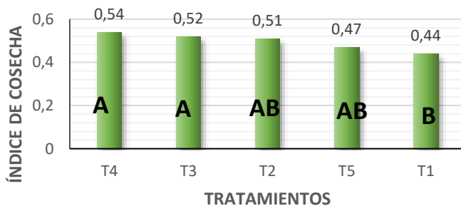
Figura 7. Prueba de Tukey al 5 % para índice de cosecha.
