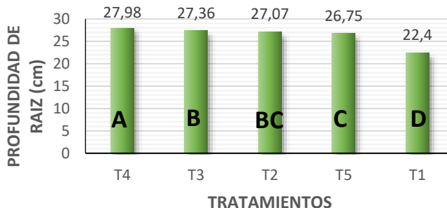
Figura 4. Prueba de Tukey al 5% para profundidad de raíz.
