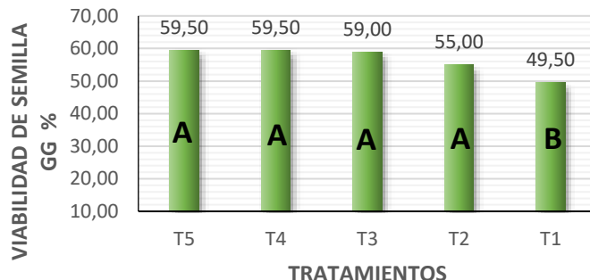
Figura 11. Prueba de Tukey al 5% para viabilidad de semilla de tamaño grande a las 16 horas de prueba.
